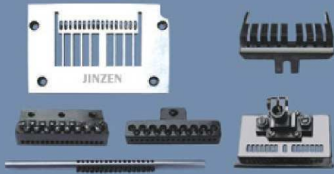
1404P 17N \times 1/8 JZ-12109
