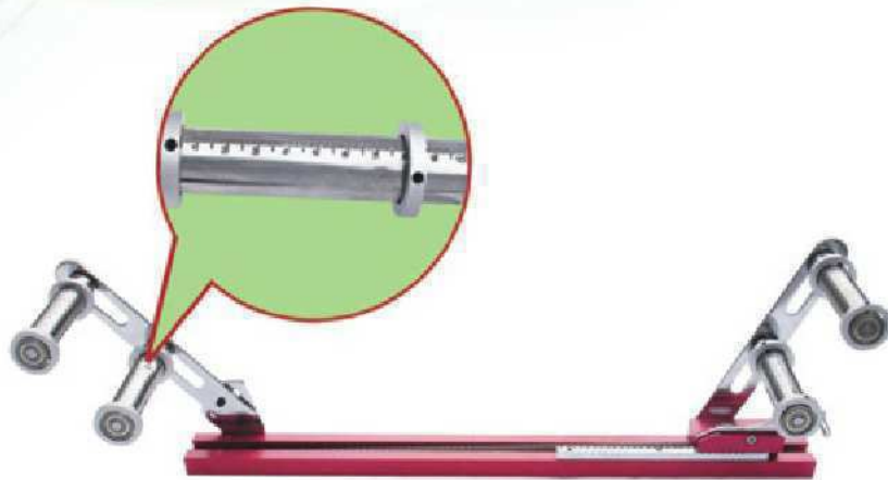
JZ-72401 特殊铝质 (带刻度) 活动啤唛架 (橡筋架) 专用于: 橡筋车 裤头车
